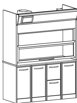
C1/A2C2S L.1610 H.2110 P.800
