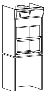
C3/R L.810 H.2110 P.800
