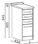
CM1-35 L.370
