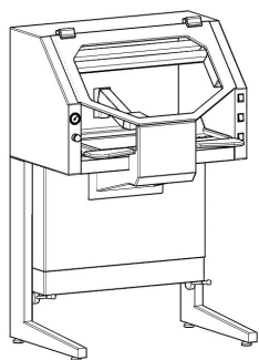
BOX CERAMICA L.840 H.1330 P.670
