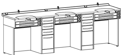
BLM303-35 L.2850
