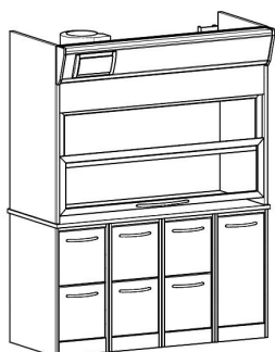
C1/C6S L.1610 H.2110 P.800
