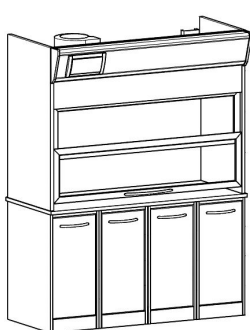
C1/A3S L.1610 H.2110 P.800
