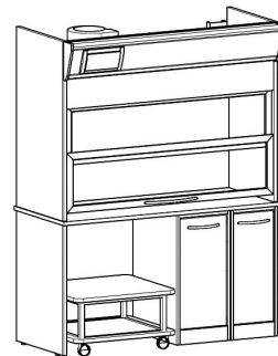
C1/RA1S L.1610 H.2110 P.800
