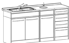
MTS2-3G/1000 L.2020 H.1000
