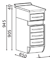
CM4/AM35 L.370
