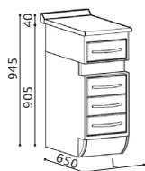
CM4/AM35 L.370
