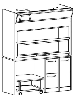
C1/RC2S L.1610 H.2110 P.800
