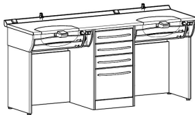
BLEK201 L.1980
